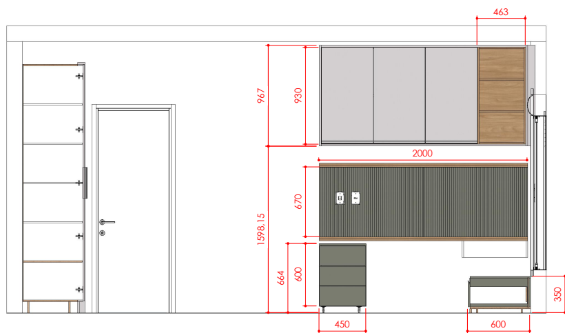
CORTE B 1:50
