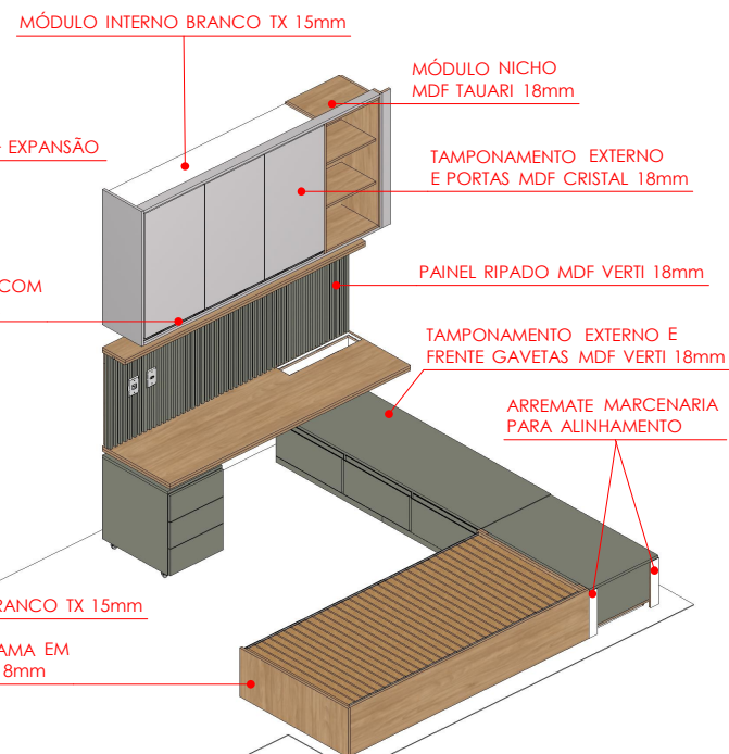
DETALHE ISOMÉTRICO 1:50
