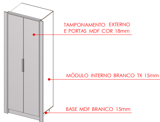
ARMÁRIO 1:50
