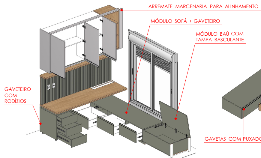
DETALHE ISOMÉTRICO 1:50
