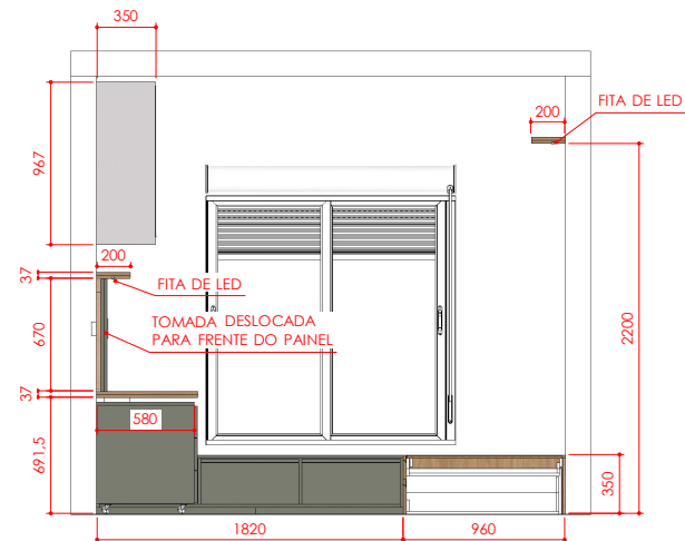
CORTE A 1:50
