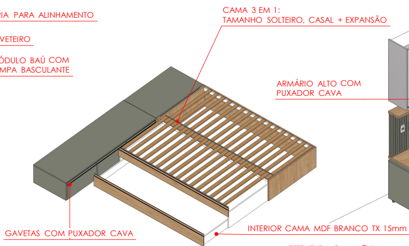
DETALHE ISOMÉTRICO 1:50
