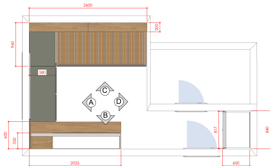
PLANTA BAIXA 1:50
