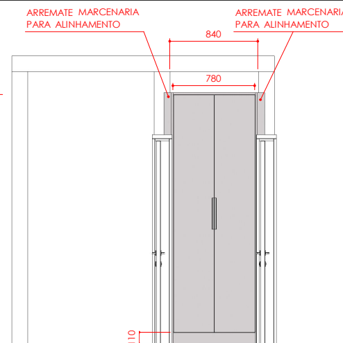
CORTE D 1:50
